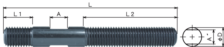
(寸法表)
